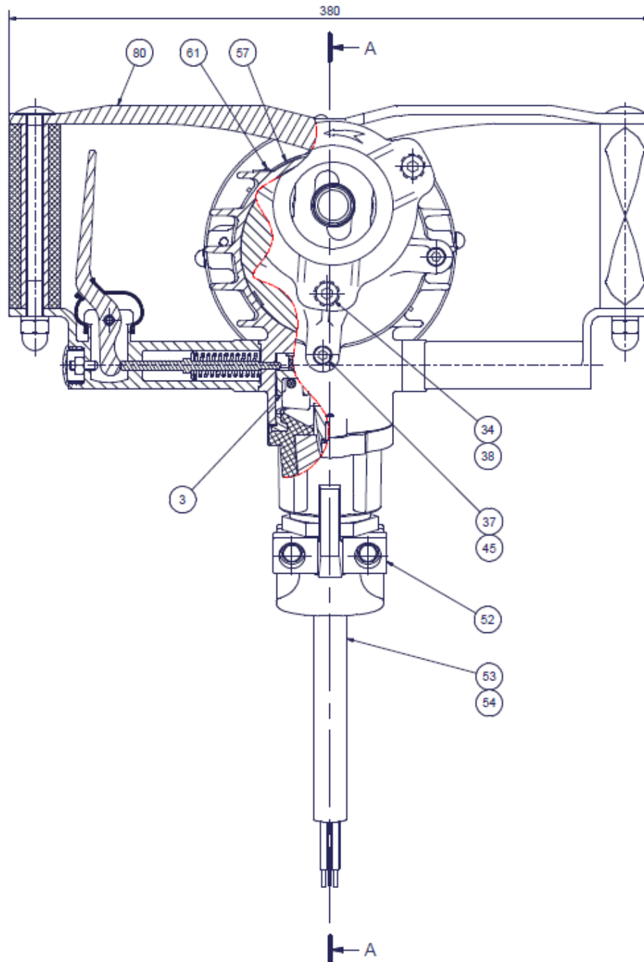
Rys.2 Wiertarka ER-6 widok z przodu
